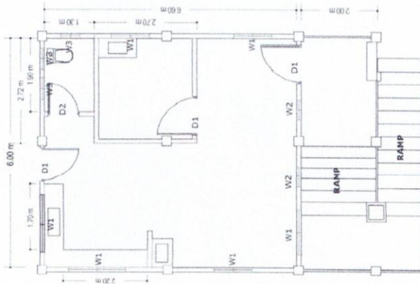
FLOOR PLAN SCALE: 1:100
