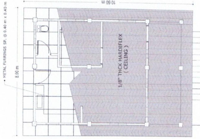
CEILING PLAN SCALE: 1:100
