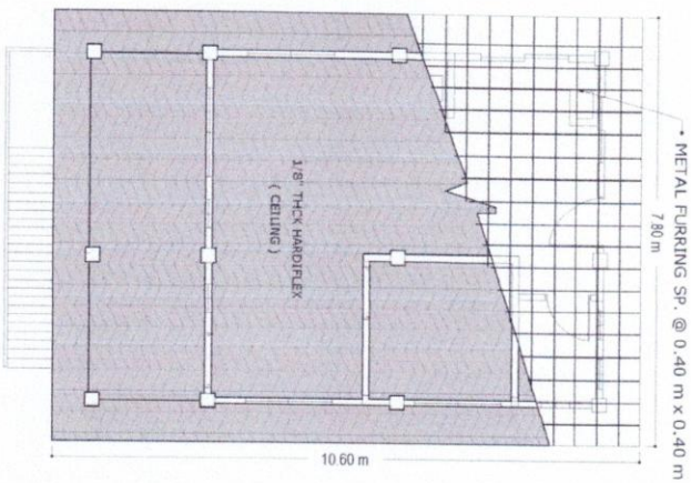
CEILING PLAN SCALE: 1:100
