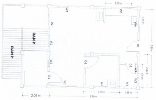
FLOOR PLAN SCALE: 1:100
