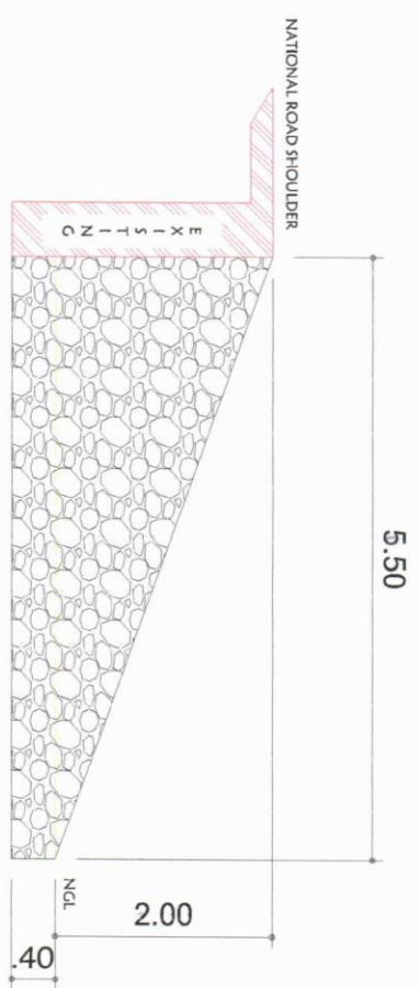
ELEVATION
